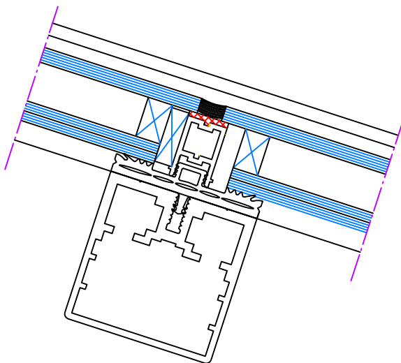
giunzione delle lastre con fessura siliconata
